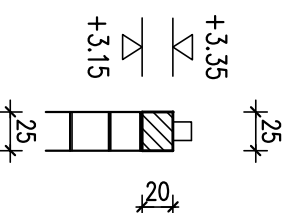
7-7 METSZET
