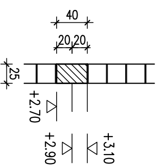
5-5 METSZET
