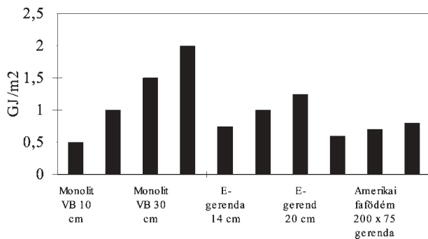
8. ábra. A födémek beépített energiája (GJ/m²)
