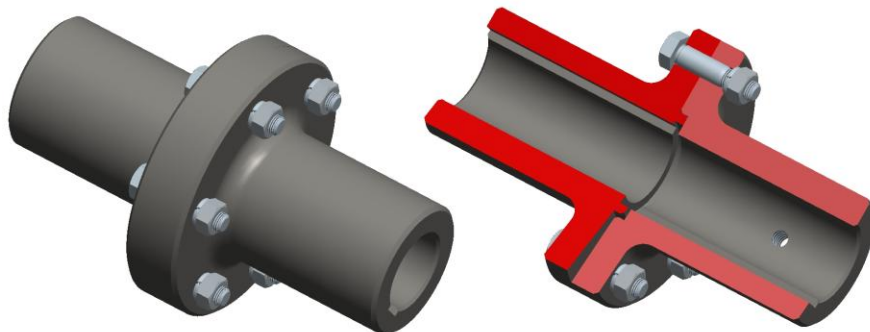
1. ábra: Az alakzáró tárcsás tengelykapcsoló felépítése, tengelyek nélkül
