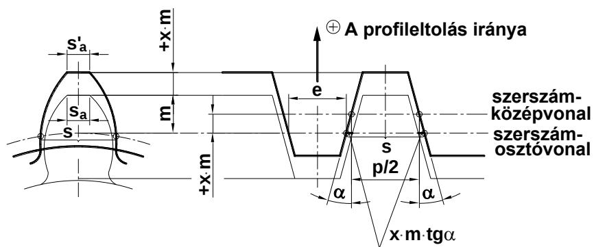
A profileltolás hatása pozitív profileltolás esetén
