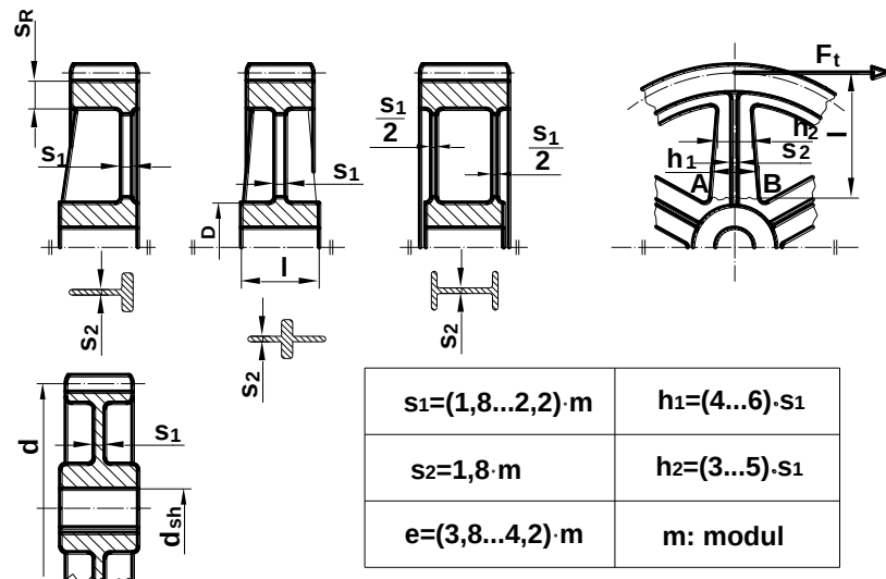
Tárcsás fogaskerék és bordákkal merevített fogaskerekek
