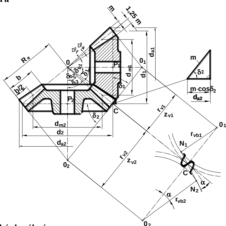
Egymással kapcsolódó kúpkerékpár
