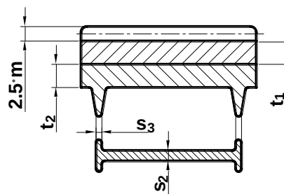
Tömbfogaskerék
