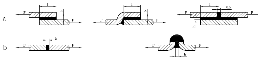
Átlapolt és hevederes forrasztott kötés
