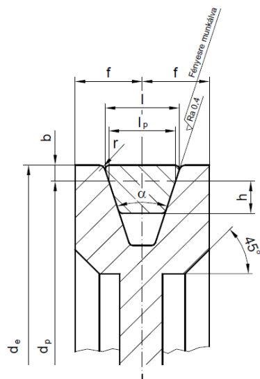
Az ékszíjtárca fő méretei
