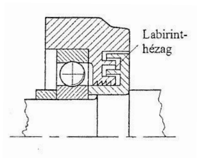
Labirinttömítés mélyhornyú golyóscsapággal
