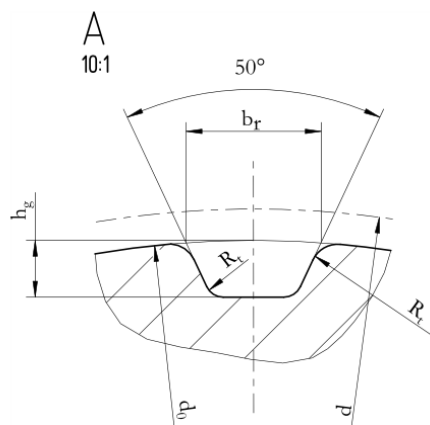
Fogárokprofil DIN 7721-10 T5x20 SE2 Fogasszíf fogárokprofil
