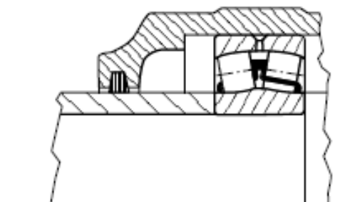
Nemez tömítés beállós görgős csapággal
