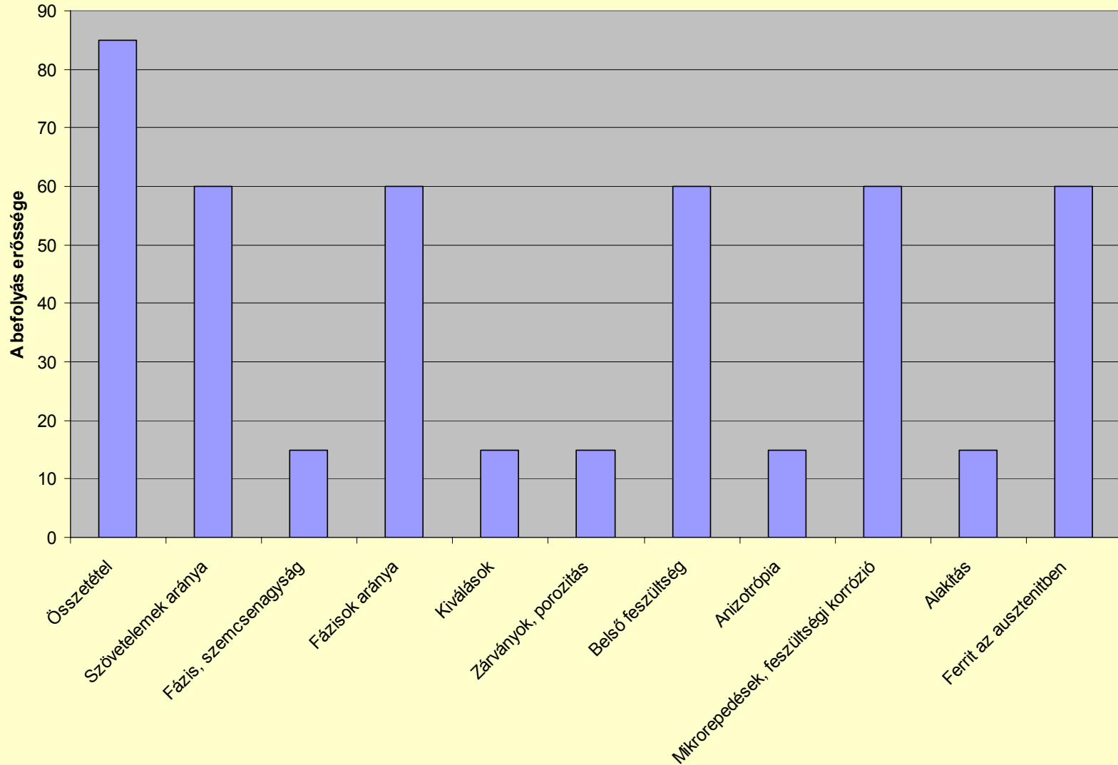
Az anyagtulajdonságok és a vezetőképesség összefüggése
