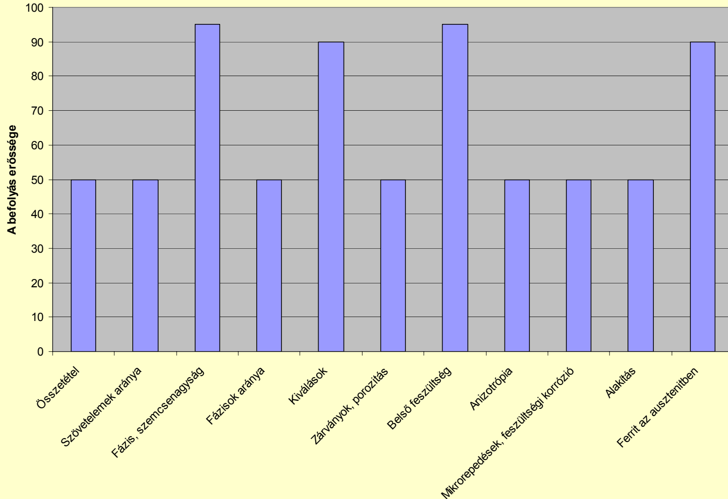
Az anyagjellemzők és a mágneses permeabilitás összefüggése
