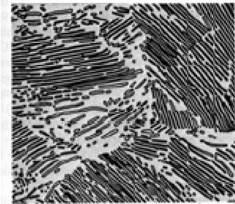
Fe-C eutektoid
