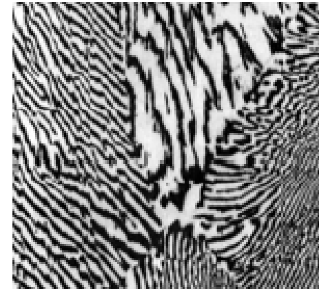
Pb-Sn eutektikum
