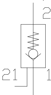
Vezérelt visszacsapó szelep
