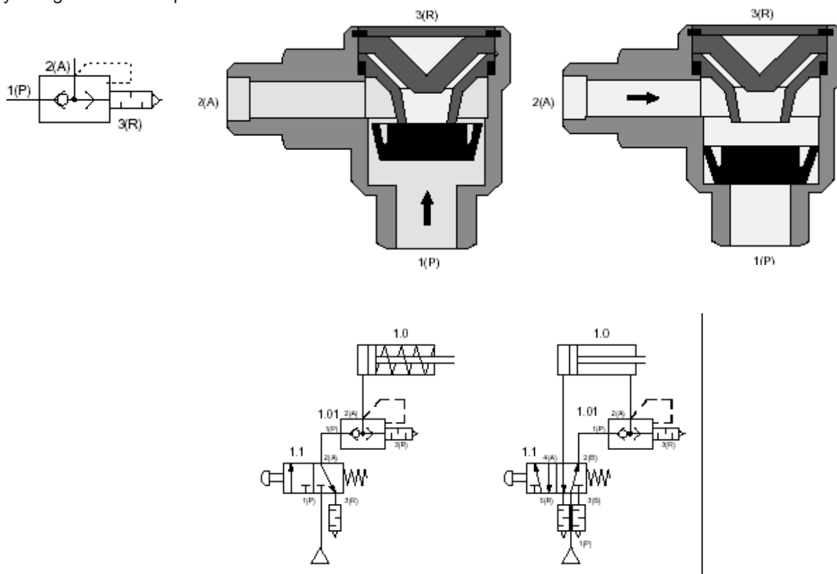
Gyorslégtelenítő szelep
