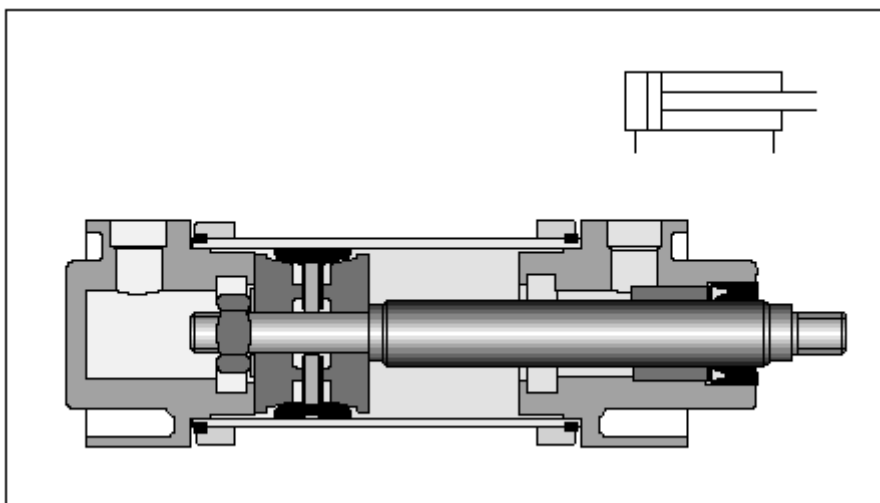
Kettősműködtetésű munkahenger
