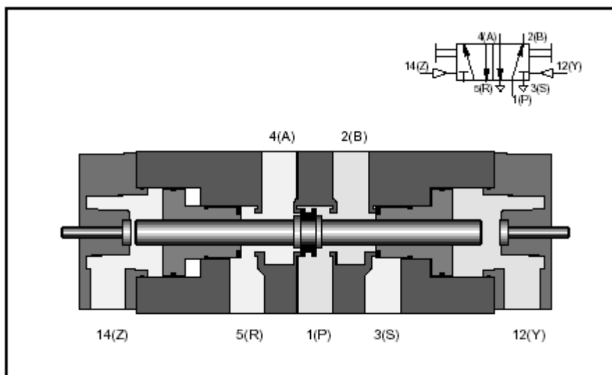
5/2-es útszelep (lebegő középállás)
