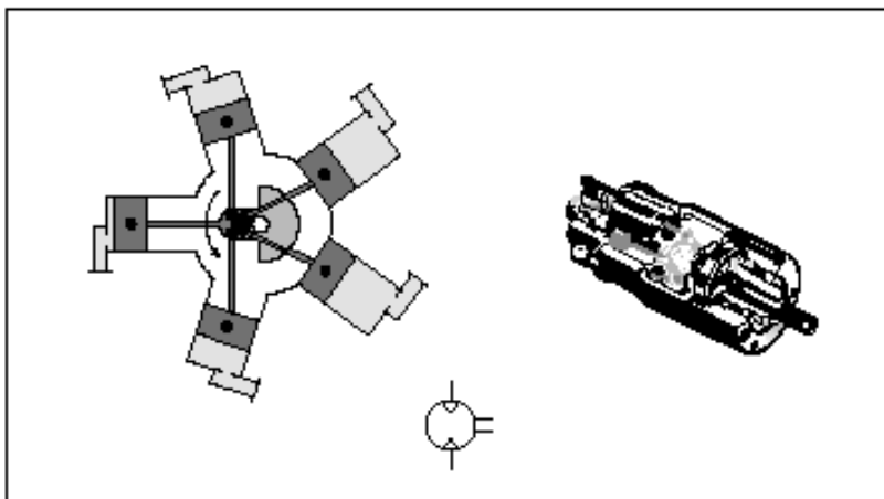
Radiáldugattyús motor
