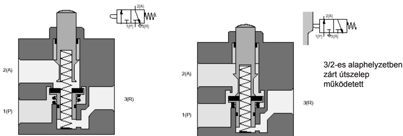
3/2-es alaphelyzetben zárt útszelep
