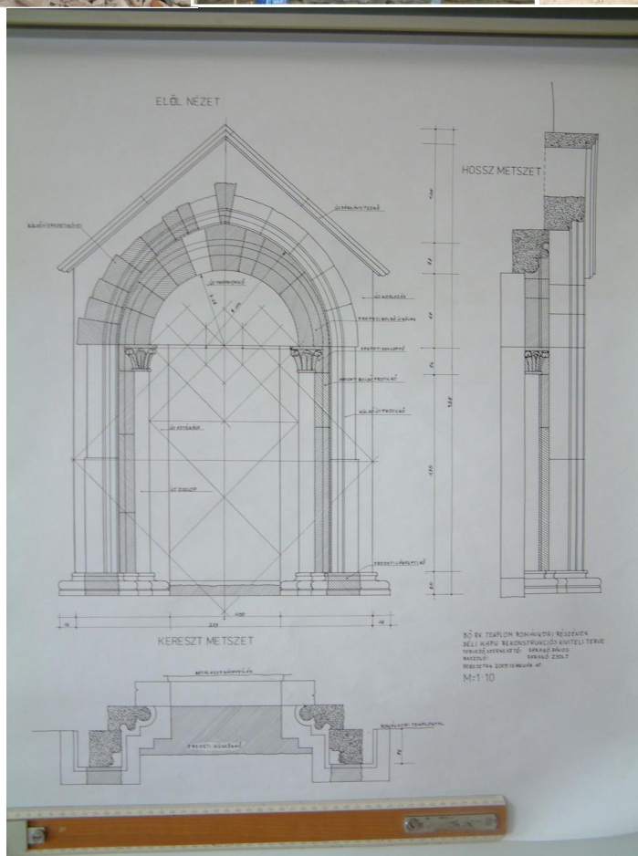
A kapu rekonstrukciós tervei
