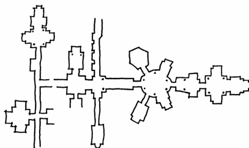
A római Via Latina alatti cubiculum-sor alaprajza.
