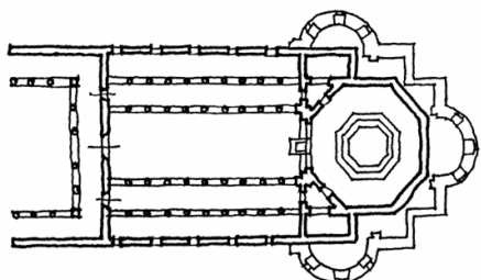
Betlehem , Jézus születése bazilika (eredeti és átépített állapot), alaprajz.
