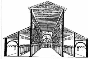
Róma, S. Pietro Vecchio bazilika (324-337), alaprajz, metszet, rekonstruált tömegvázlat.
