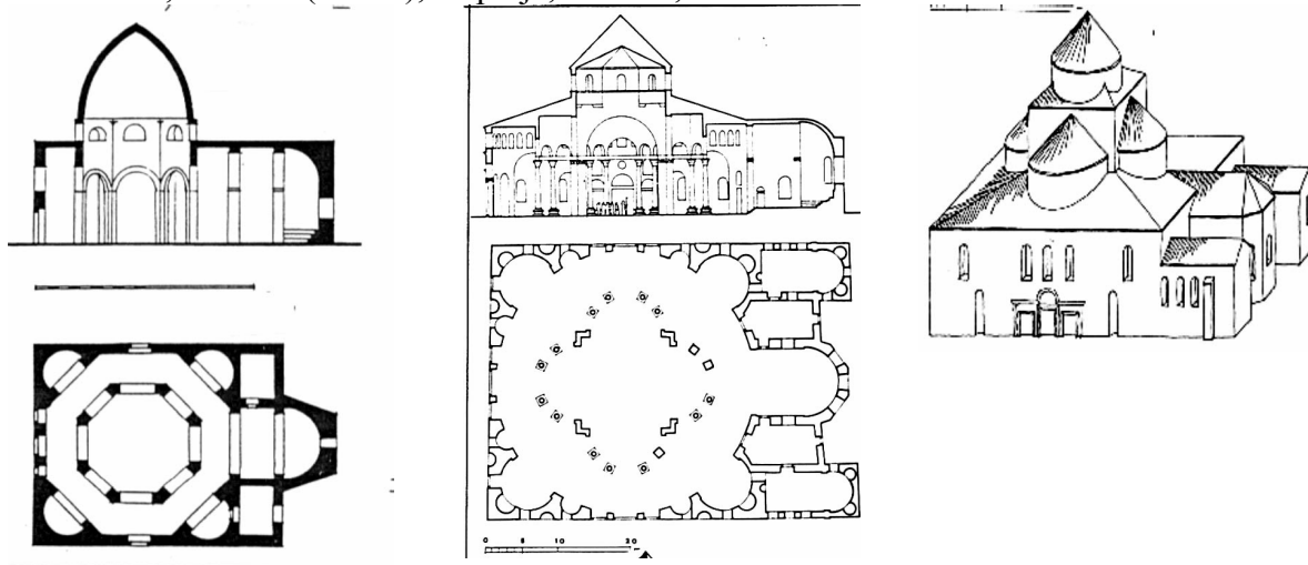
Eszra, Sz. György templom (515), alaprajz, metszet.
