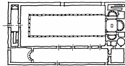
Deir-el-Abiad, kolostortemplom, alaprajz.
