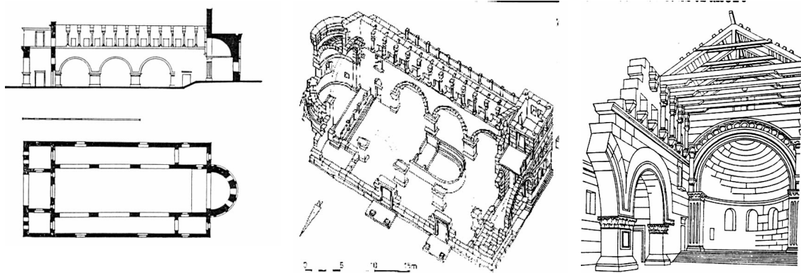
Qalb-Luzeh , püspöki székesegyház. Alaprajz, metszet, axonometrikus metszet, belső rekonstrukció.
