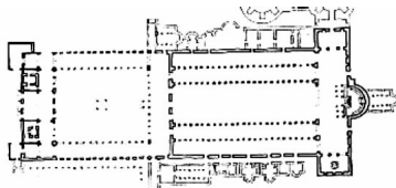
Róma, S. Giovanni in Laterano (313-320), alaprajz.
