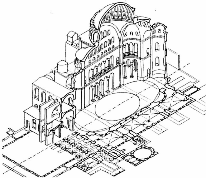
Konstantinápoly, Hagia Szophia templom, axonometrikus metszet.
