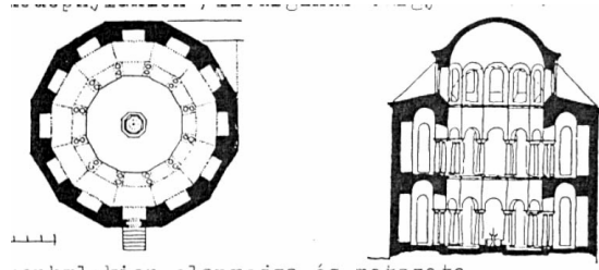
Konstantinápoly, Hagia Szophia templom, a Szkeuophylakion alaprajza és metszete.
