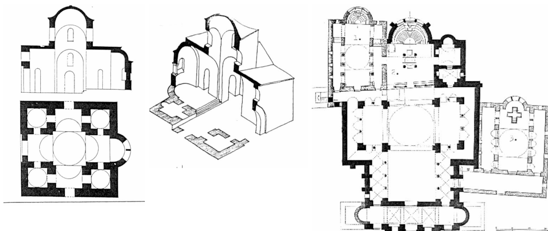
Thesszaloniké, Hosziosz David, a Latomosz kolostor kápolnája: alaprajz, metszet, axonometrikus metszet.
