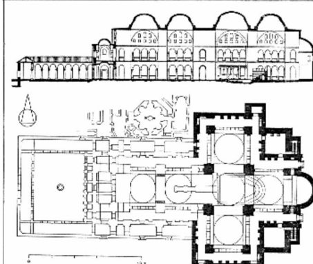
Epheszosz, Sz. János templom (VI. sz. eleje), alaprajz, metszet.
