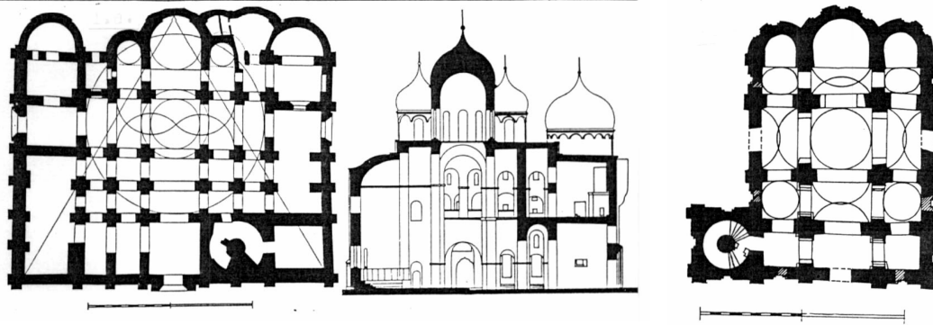
Novgorod , Sz. Szófia székesegyház (1045-1050), alaprajz, metszet.
