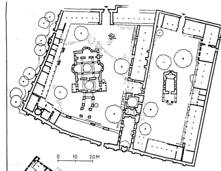
Bacskovo, kolostor (XI. sz., 1604), alaprajz.
