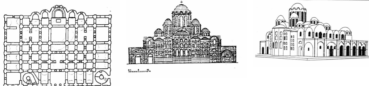
Kijev, Sz. Szófia székesegyház (1037-1067), alaprajz, keleti homlokzat, tömegvázlat.
