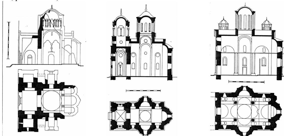
Dzsurdzsevi-Sztubovi (1170), templom, alaprajz, metszet.
