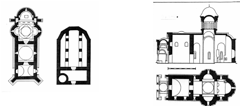
Keleti és nyugati hatás ötvöződése: Voronet , kolostortemplom (1457-1504), Cozia , kolostortemplom (1386), alaprajz, metszet. Cîmpulung , bazilika (XIII-XIV. sz.), alaprajz.
