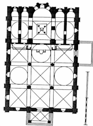
Moszkva, Uszpenszkij székesegyház (1326-1333. ill. 1467-1479), alaprajz, metszet.
