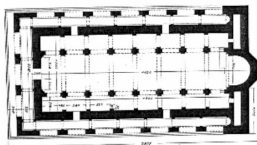
Dvin, székesegyház II. periódus (VI. sz.), alaprajz.
