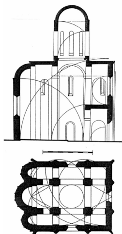
Vlagyimir, Sz.Demeter templom (1094-1097), alaprajz, metszet.
