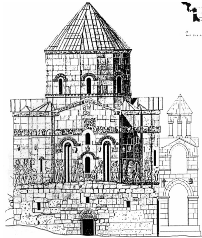
Aghtamar , Sz. Kereszt templom (915-921), alaprajz, nyugati homlokzat.
