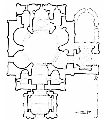
Nikoremda , (1010-1014), templom, alaprajz.
