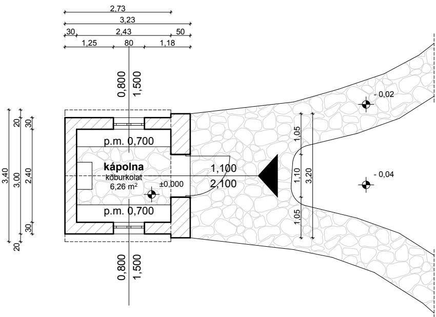
2. Kápolna alaprajza m 1:100
