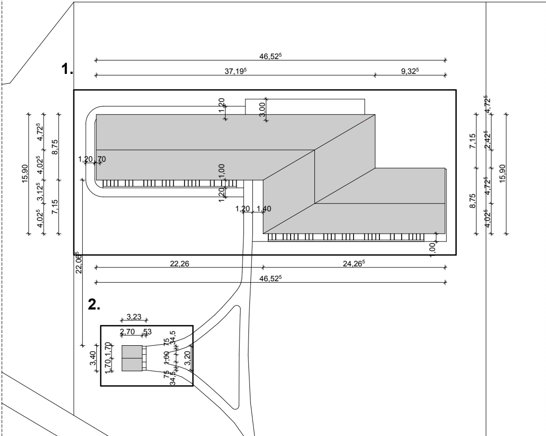
Helyszínrajz m 1:500
