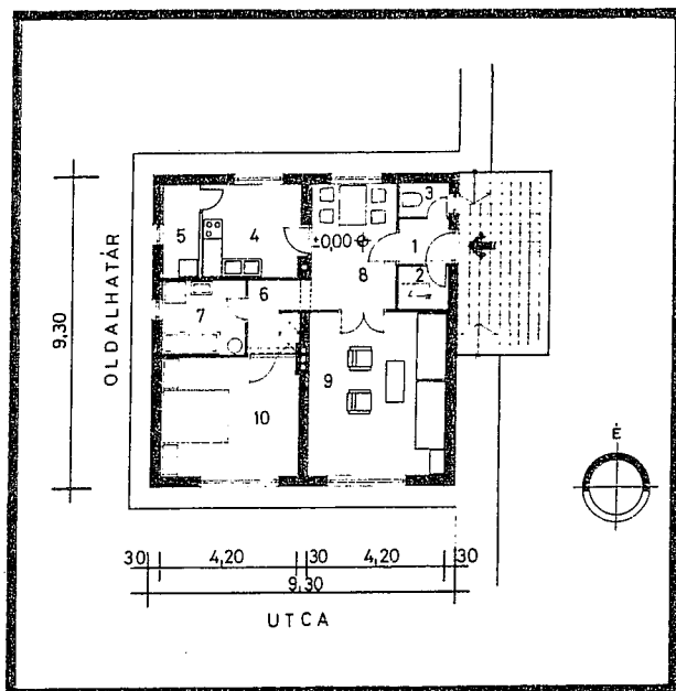
Sátortetős változat CS 00 H 10 AV S
