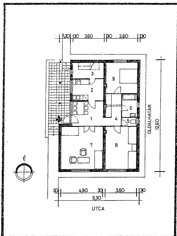
Utcaira merőleges gerincű nyeregtetővel CS 00 H 15 A M
