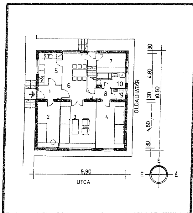
Sátortetős változat CS 00 H 14 A S
