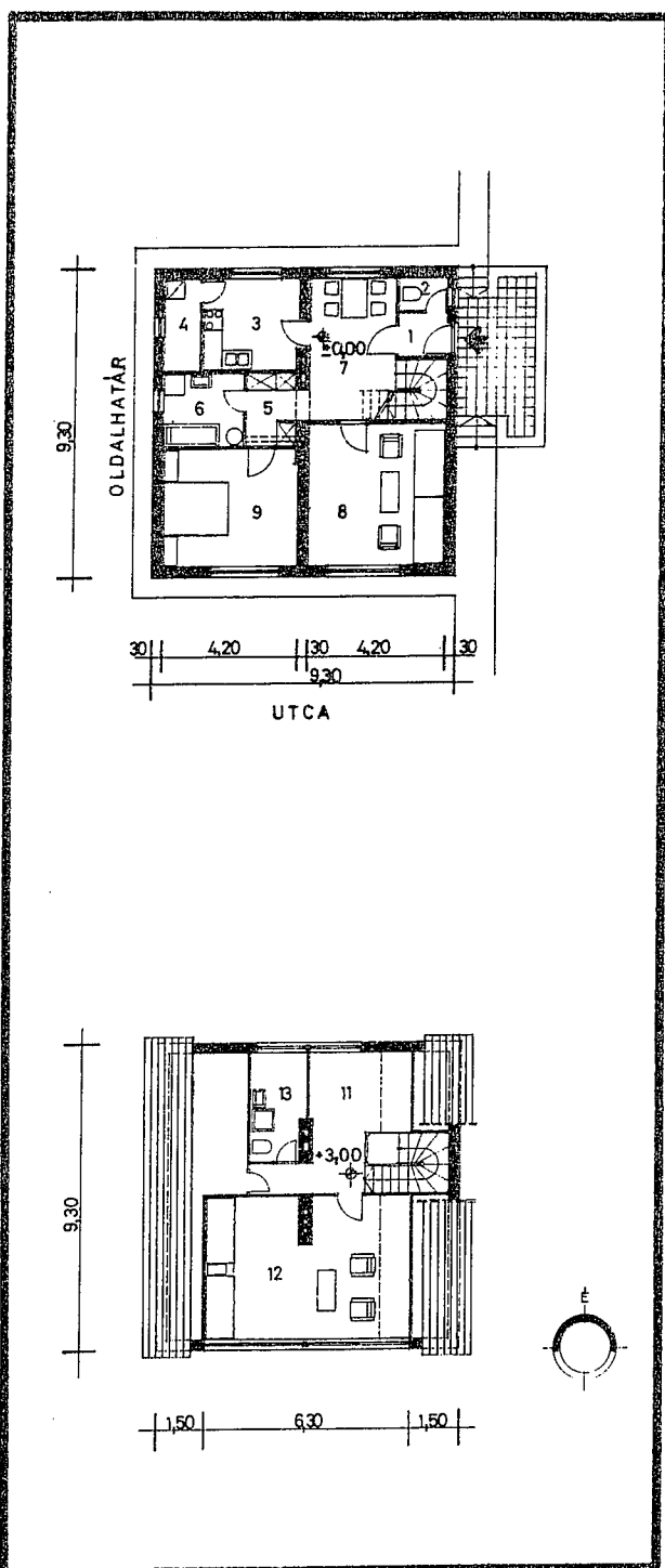
Utca-ra merőleges gerincű nyeregtetővel CS 00 H 10 TV M
