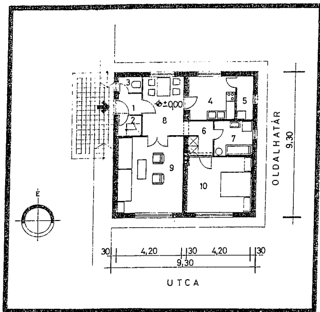
Sátortetős változat CS 00 H 10 A S
