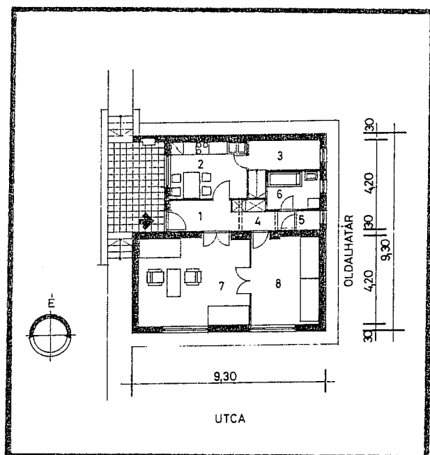
Sátortetős változat CS 00 H 11 A S
