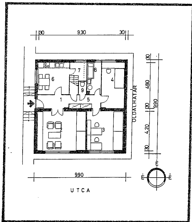
Utcával párhuzamos gerincű nyeregtetővel CS 00 H 16 A P
