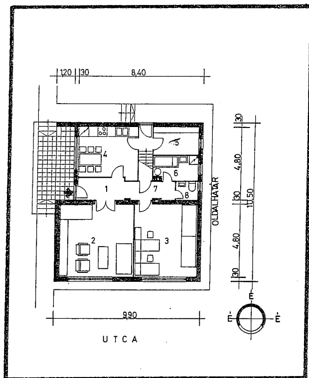
Sátortetős változat
