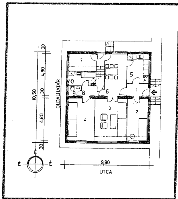
Sátortetős változat
