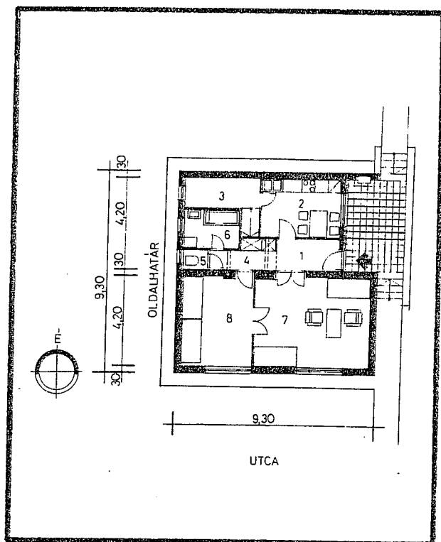
Sátortetős változat CS 00 H 11 AV S
