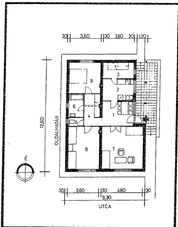
Utcára merőleges gerincű nyeregtetővel CS 00 H 15 AV M
