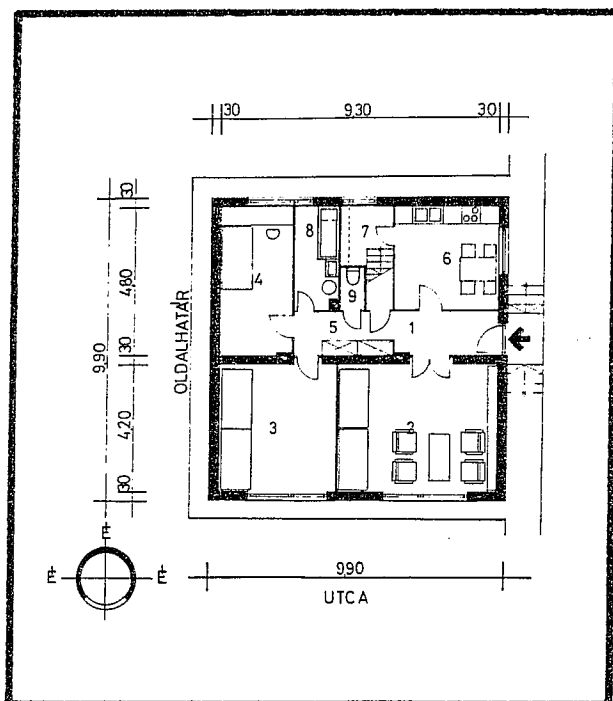
Utcával párhuzamos gerincű nyeregtetővel CS 00 H 16 AV P
