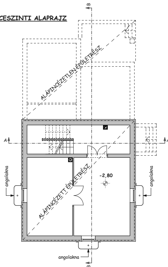
FÖLDSZINTI ALAPRAJZ
