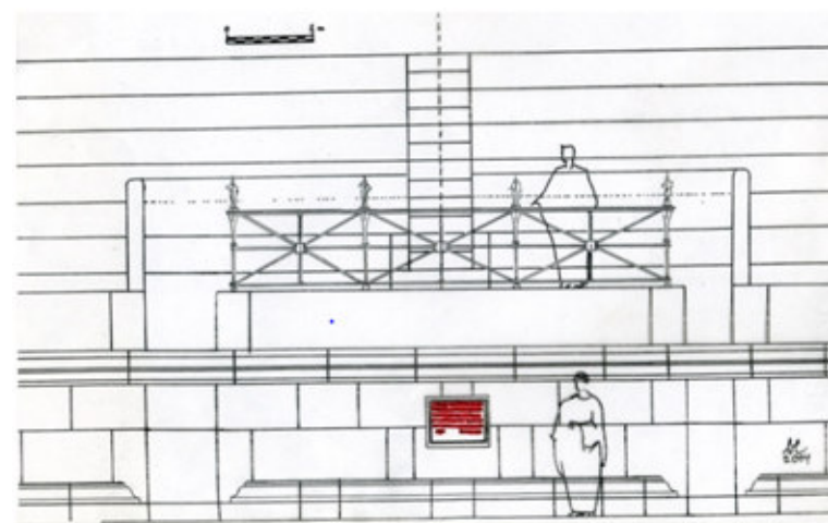
85. ábra: A brigetiói podium-felirat lehetséges elhelyezkedése az egykori podium-falban (rajz: Borhy László)
