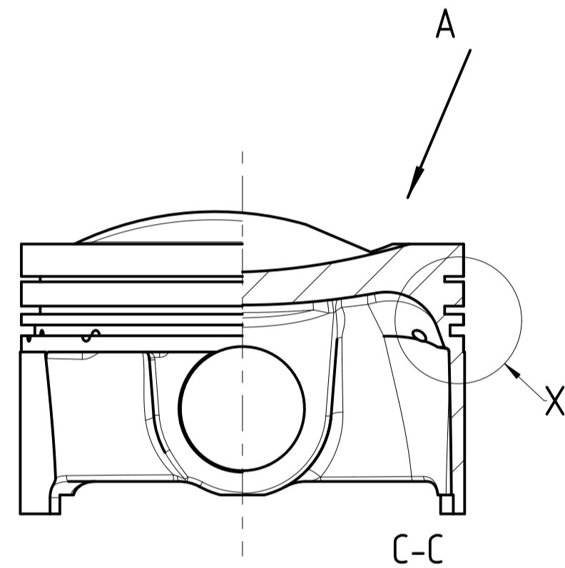
Félnézet - félmetszet - Half Cross Section
