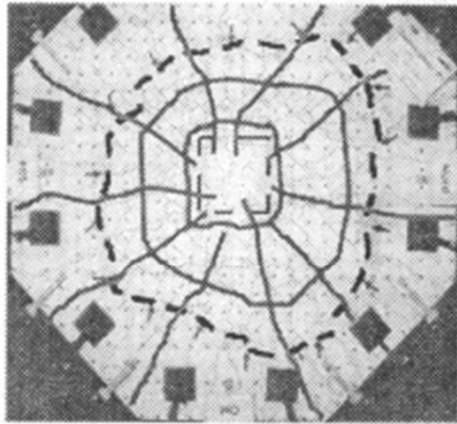
Felső repedési kép
