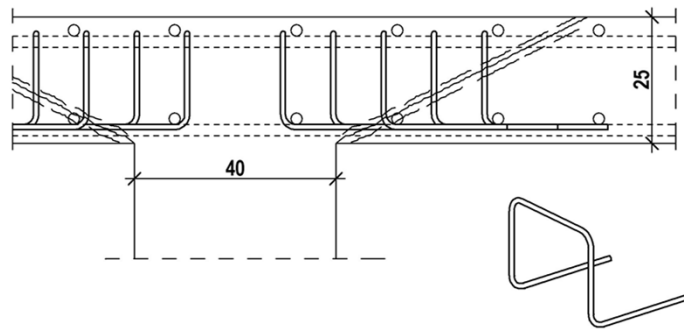
metszet
