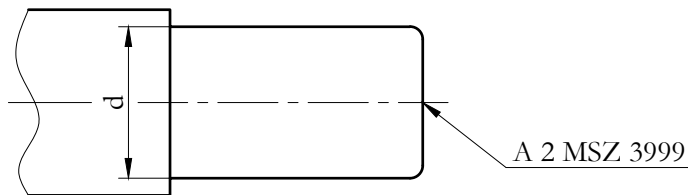
4.10. ábra. Központfurat jelölése
