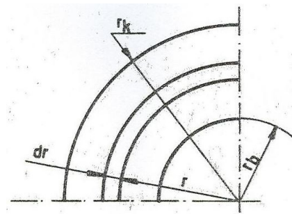
5.29. ábra. A közepes sugár értelmezése dörzstárcsás tengelykapcsolónál
