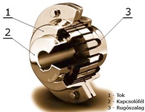
5.21. ábra. Bibby tengelykapcsoló
