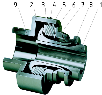
5.31. ábra. Lemezes dörzskapcsoló
