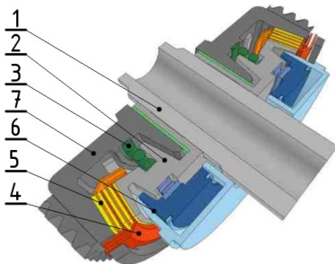
5.27. ábra. Súrlódó kúpos tengelykapcsoló
