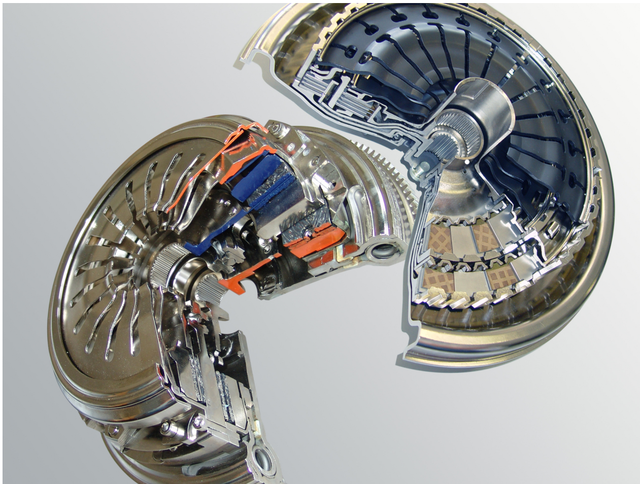
5.30. ábra. Dörzstácsás tengelykapcsolós
