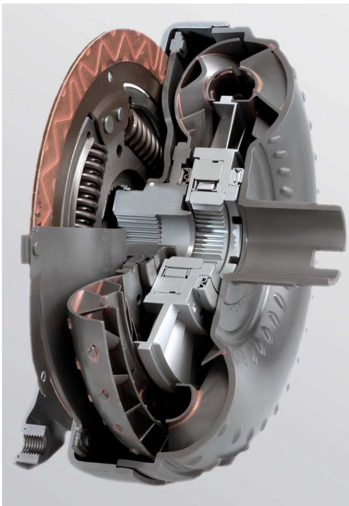
5.35. ábra. Hidrodinamikus tengelykapcsoló fényképe
