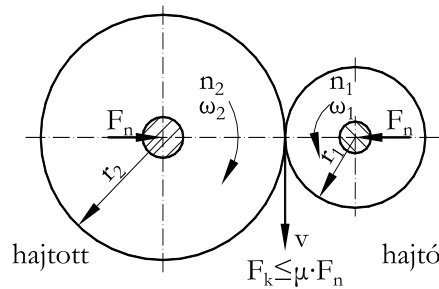
7.1. ábra. Párhuzamos tengelyű dörzshajtás elvi vázlata
