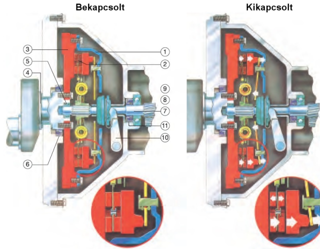
5.28. ábra. Dörzstárcsás tengelykapcsoló
