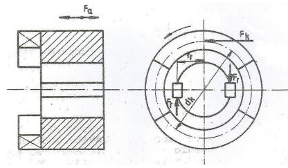
5.23. ábra. Erőhatások körmös tengelykapcsolón
