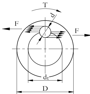
2.29. ábra. Biztosítószege ható erők
