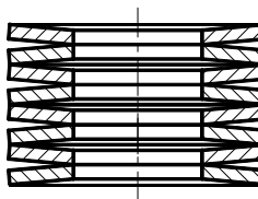
9.6. ábra. Belleville-féle tányérrugó
