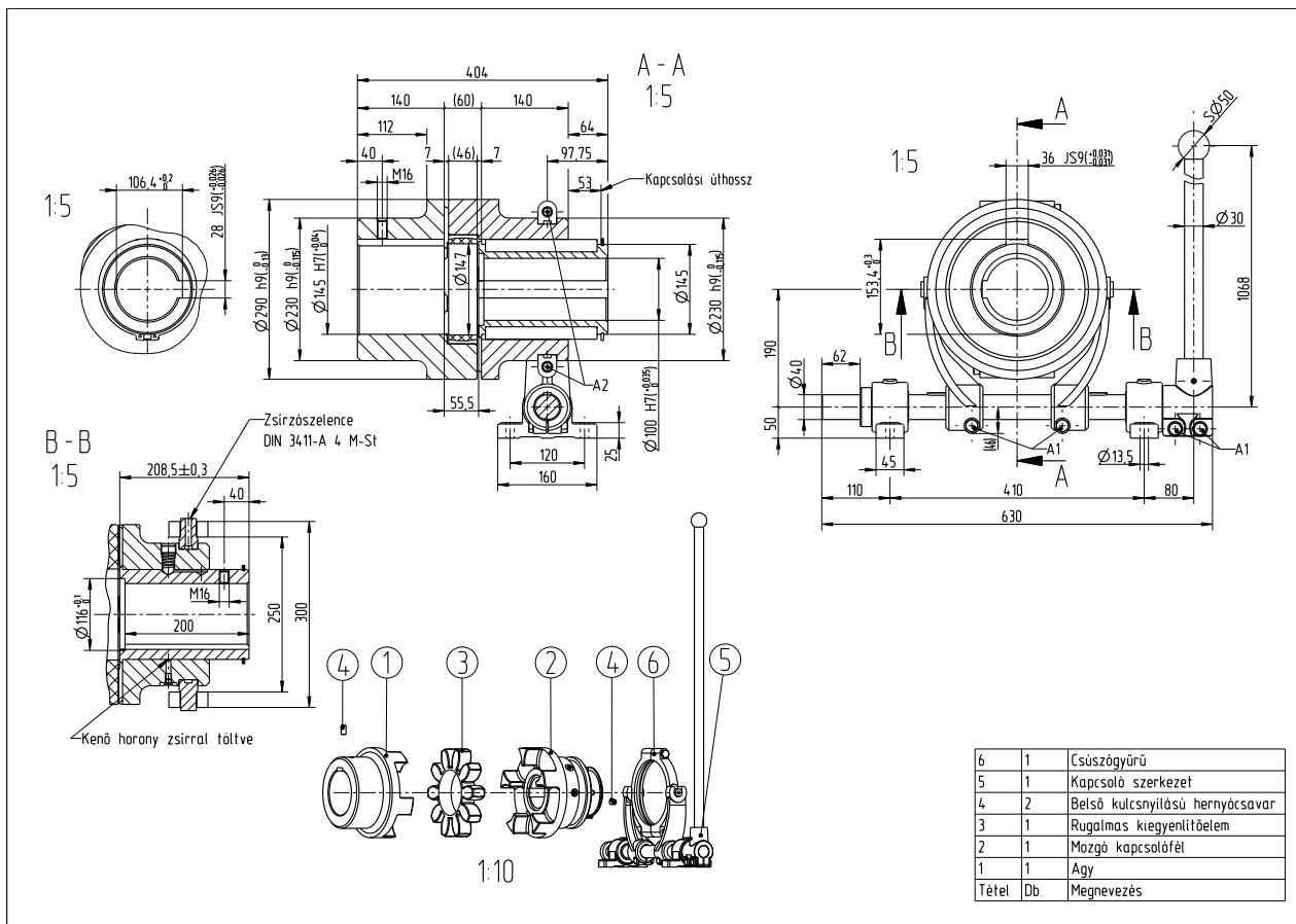
5.22. ábra. Oldható körmös tengelykapcsoló összeállítási rajza
