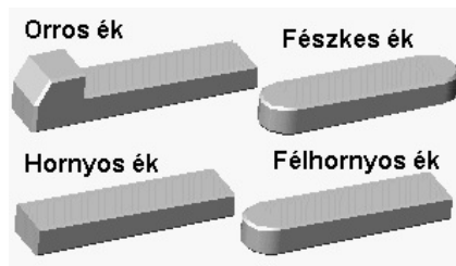
2.34. ábra. Az ékek térhatású ábrái
