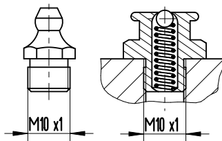
6.8. ábra. Zsírógombok
