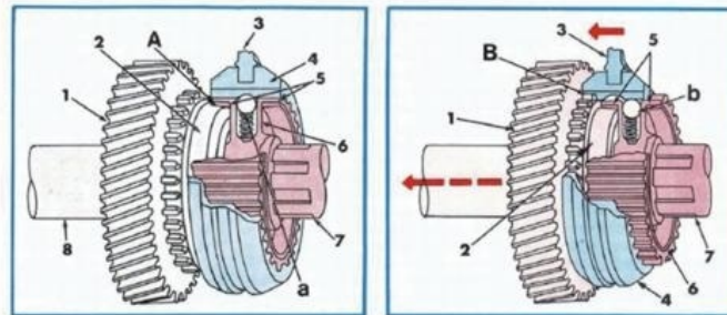
5.25. ábra. Szinkronkapcsoló 3D-s modellje
