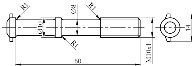
2.15. ábra. Változó keresztmetszetű csavar
