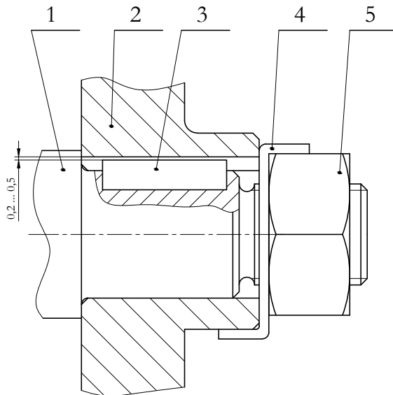
2.43. ábra. Csavaranyával való rögzítés menetes végcsonon
