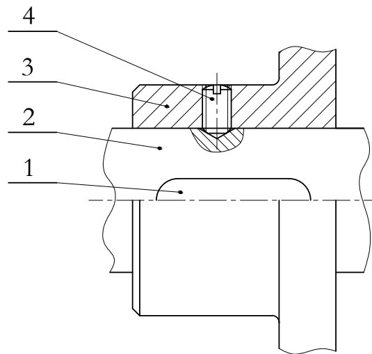
2.44. ábra. Tárcsa tengelyirányú biztosítása kúpos végű hernyócsavarral
