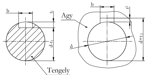
2.40. ábra. A reteszhorony méretei
