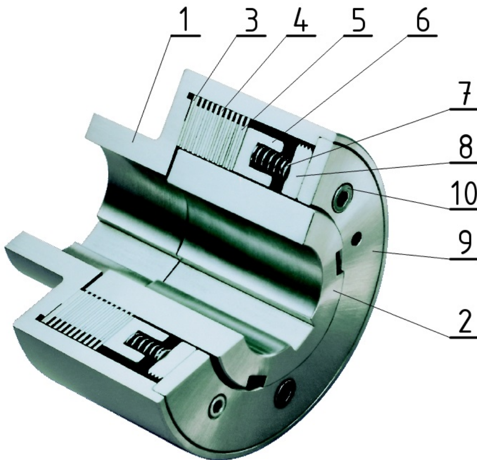
5.33. ábra. Súrlódó lemezes biztonsági tengelykapcsoló 3D-s modellje
