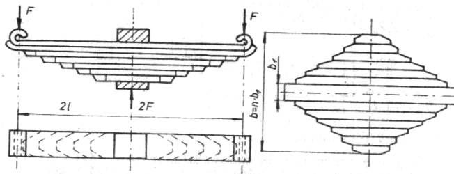
9.4. ábra. Réteges lemeZRugó
