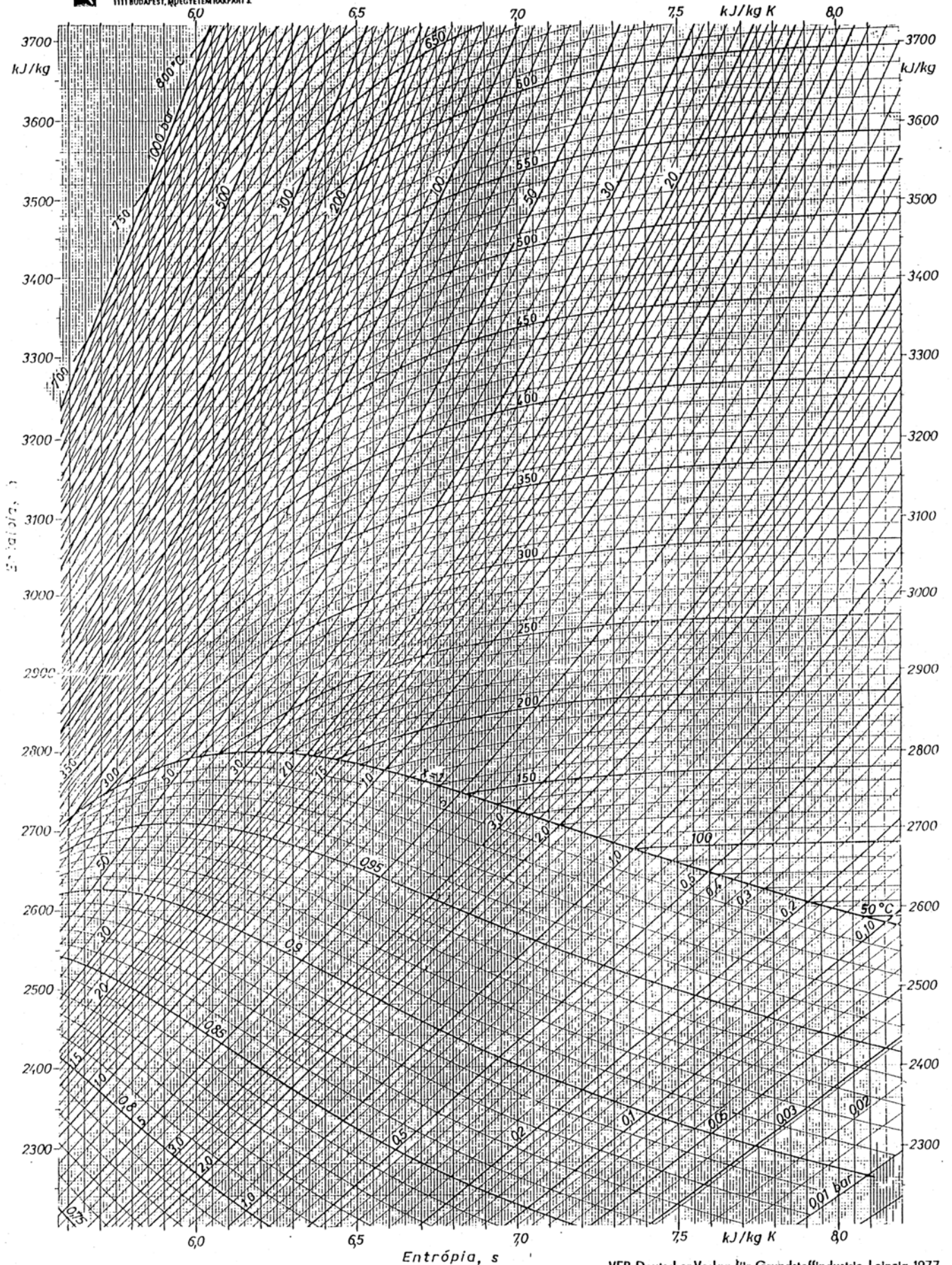
Vízgőz h-s diagramja
